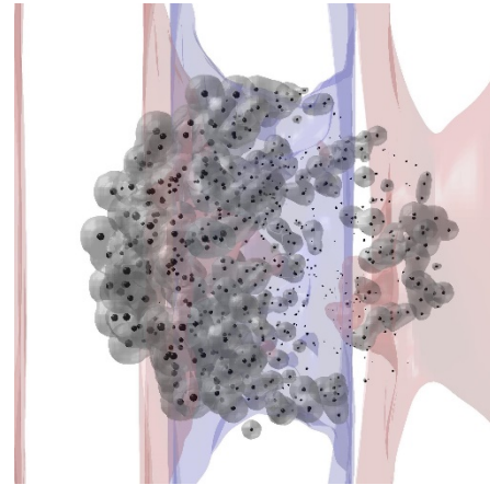
収束超音波と相互作用を行う気泡群。体積振動する気泡の表面を黒色で、高圧力場、低圧力場の等値面を赤色及び青色で、気相体積率分布の等値面を白色で示している。
